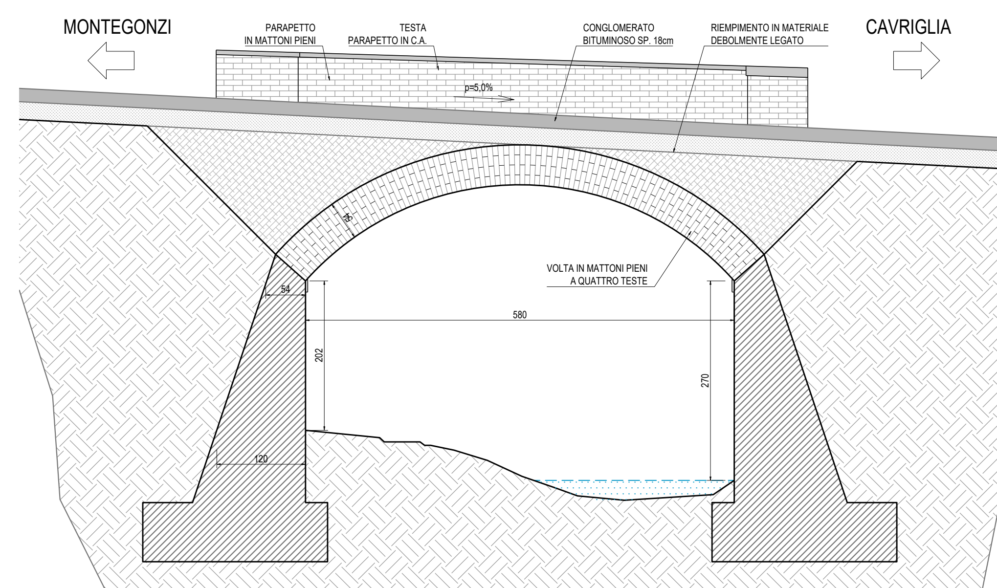
Sezione longitudinale B-B scala 1:50
