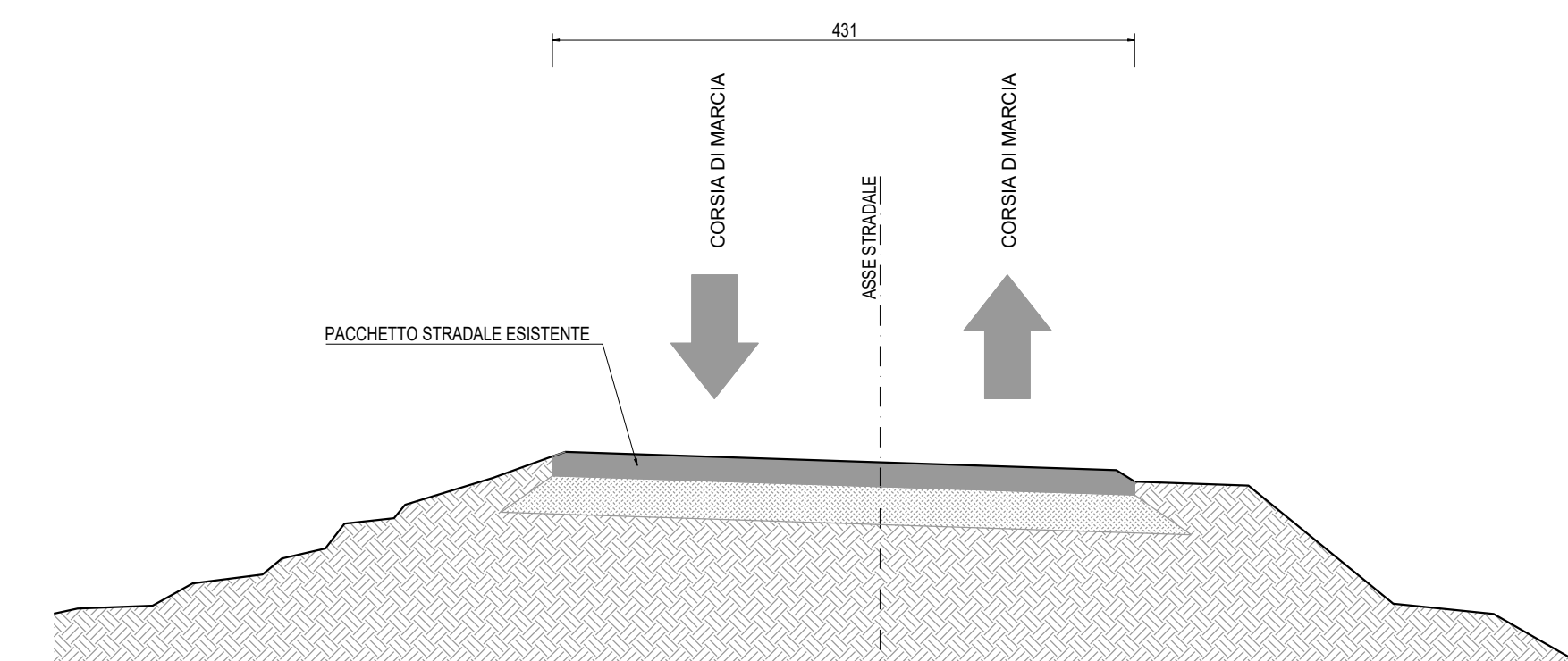
Stato di Fatto - Sezione trasversale A-A scala 1:50
