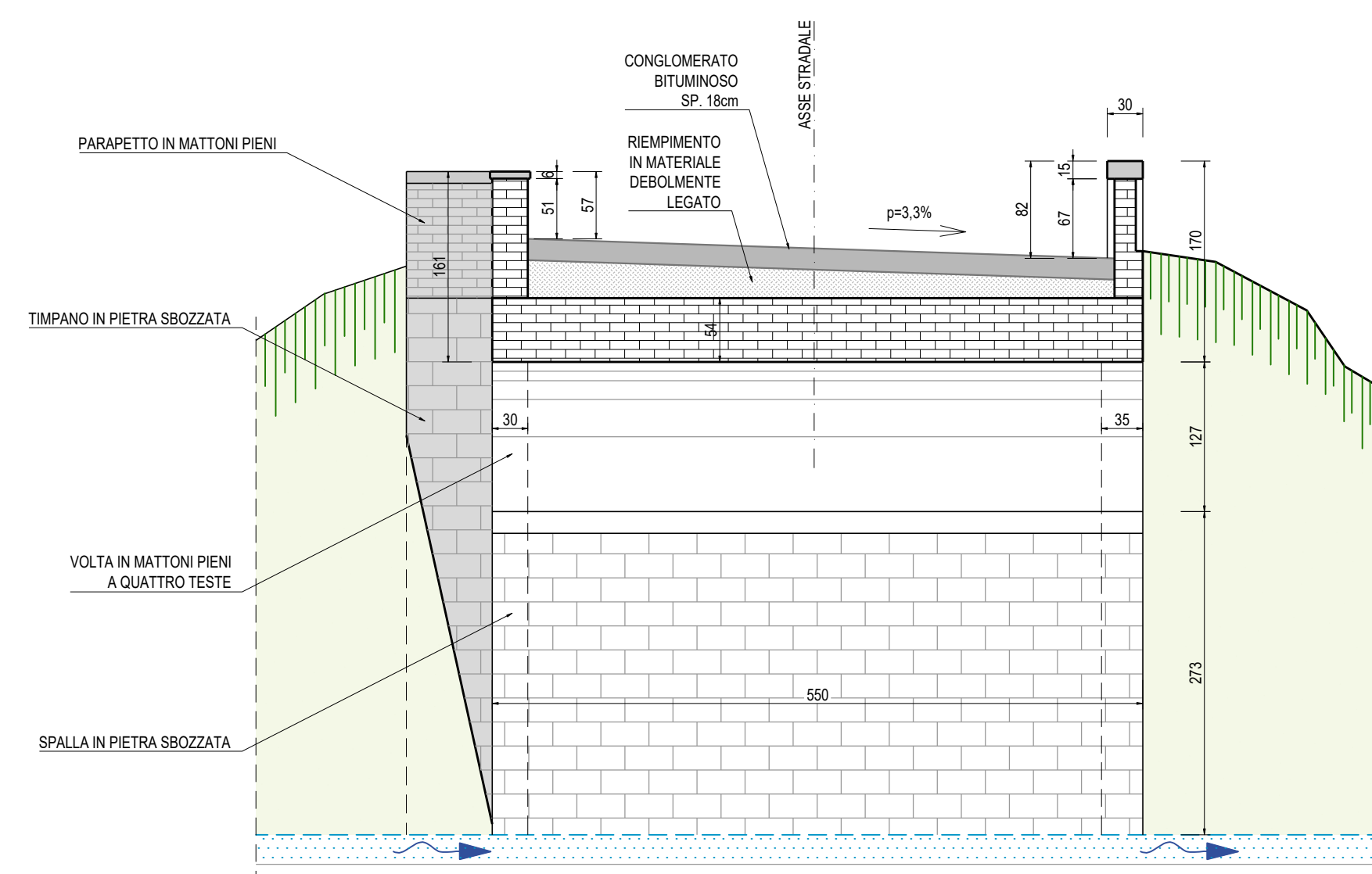
Sezione trasversale A-A scala 1:50
