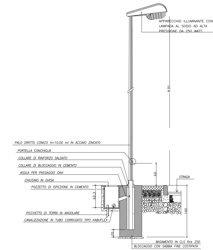
LAMPIONE TIPO "A" LAMPIONE TESTA PALO PER VIABILITA' PRINCIPALE (PALO h.f.t. = 8,00 mt.)
