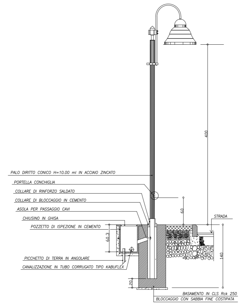
LAMPIONE TIPO "B" PUNTO LUCE PER VIABILITA' INTERNA E VERDE PUBBLICO (PALO h.f.t. = 4,00 mt.)
