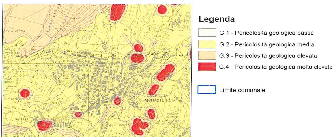
Carta delle aree a pericolosità geologica del Quadro Conoscitivo del Piano Strutturale.
